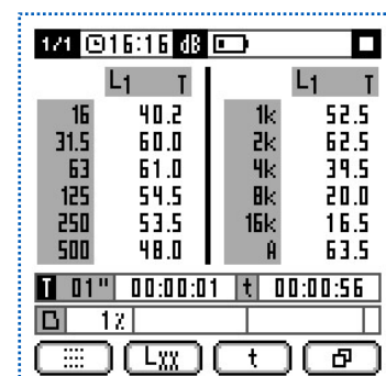
Ecrã estatístico: mostra o valor dos percentis
