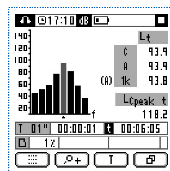
Ecrã espectral: mostra em tempo real o espectro medido
