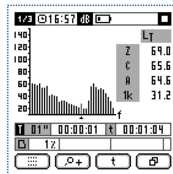
Ecrã gráfico: mostra em tempo real o espectro medido
